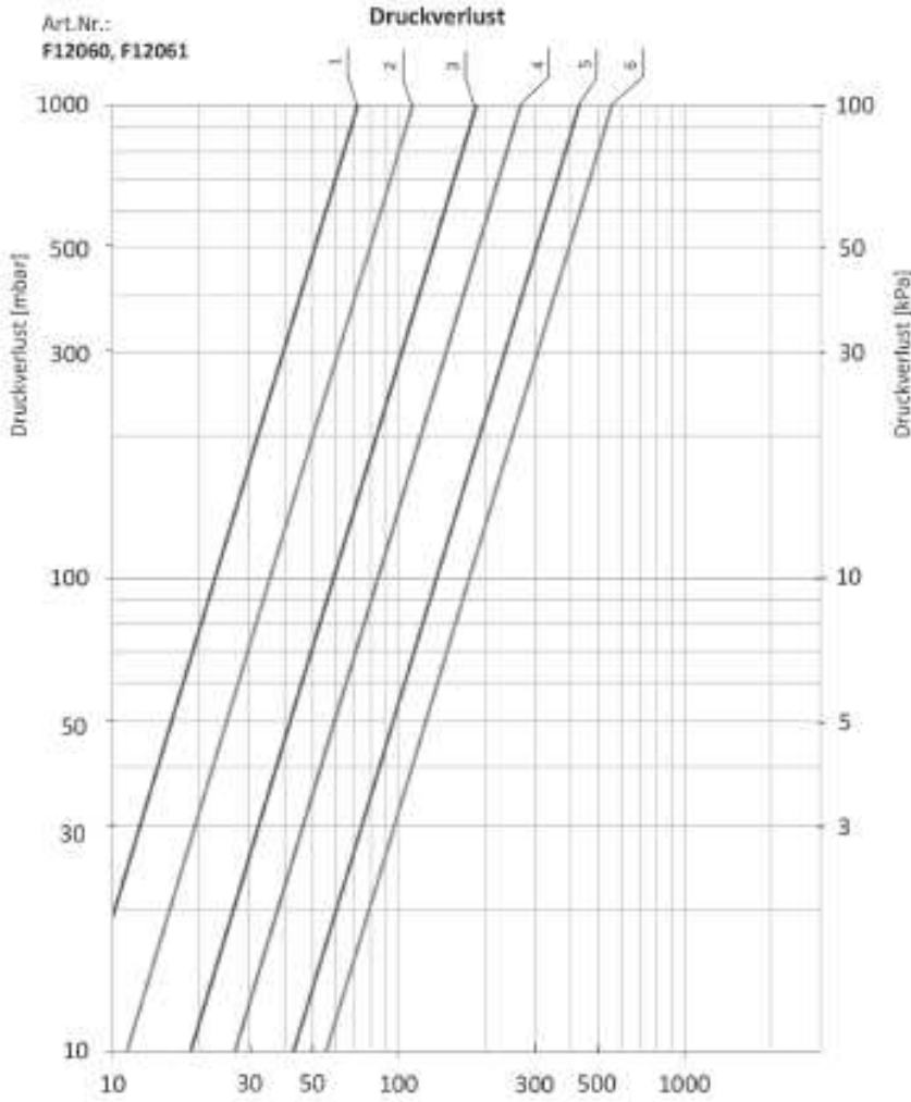
Bild 2: Druckverlustdiagramm
