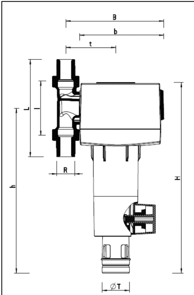
Bild 3: Baumaße Logafix Wasserfilter mit Anschlussstück
